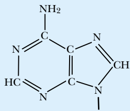
ADENOSINE
