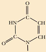
URIDINE
