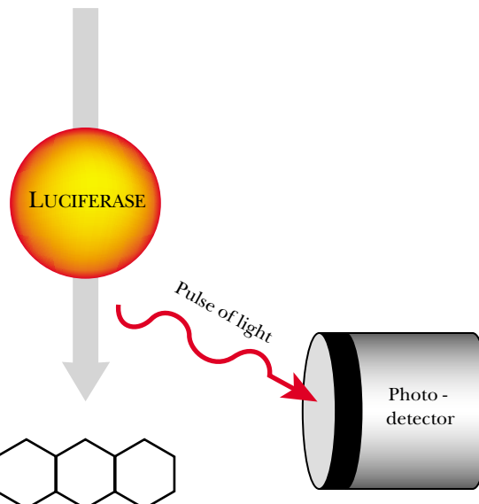
LUCIFERIN
