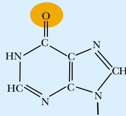
INOSINE
