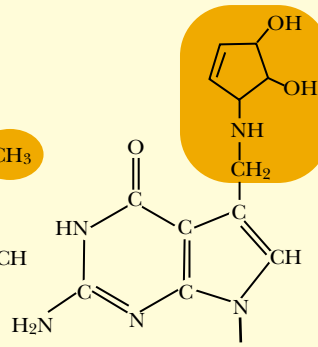
QUEUOSINE (Q)
